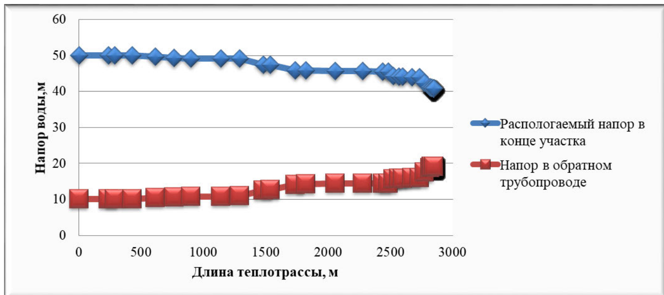
Рисунок 2.5 – Пьезометрический график тепловой сети котельной МУП «Баганский коммунальщик» с. Савкино по магистральному выводу
