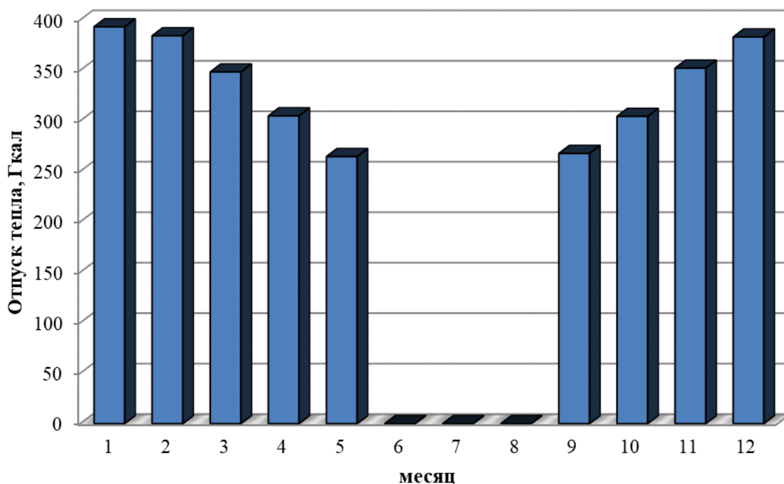
Рисунок 1.2 – Оптимальный температурный график отпуса тепловой энергии для котельной МУП «Баганский коммунальщик» Савкинского сельсовета
