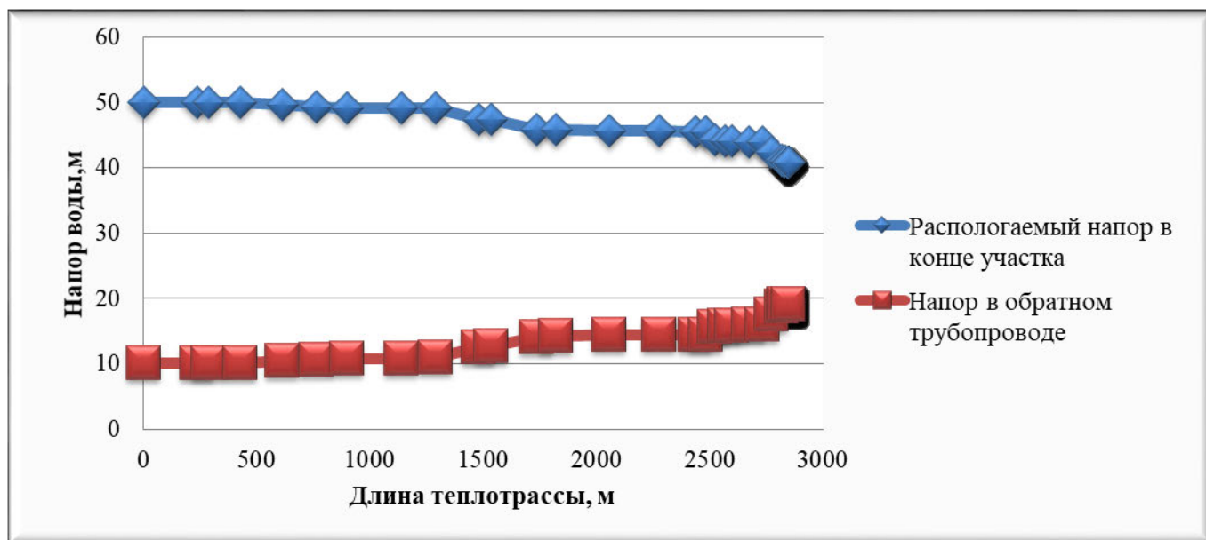
Рисунок 2.4 – Пьезометрический график тепловой сети котельной МУП «Баганский коммунальщик» с. Савкино по магистральному выводу
