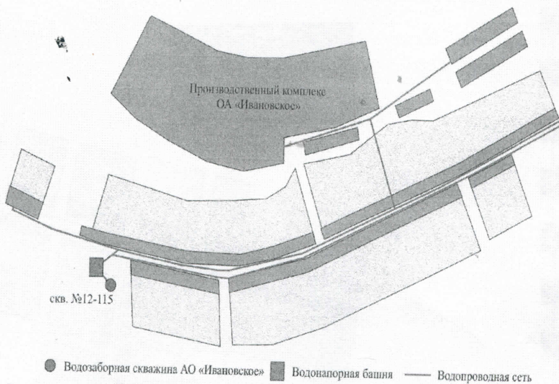
Рисунок 7.2.2. План территории АО «Ивановское» с наложением сетей водоснабжения и водоотведения (с. Подольск)
