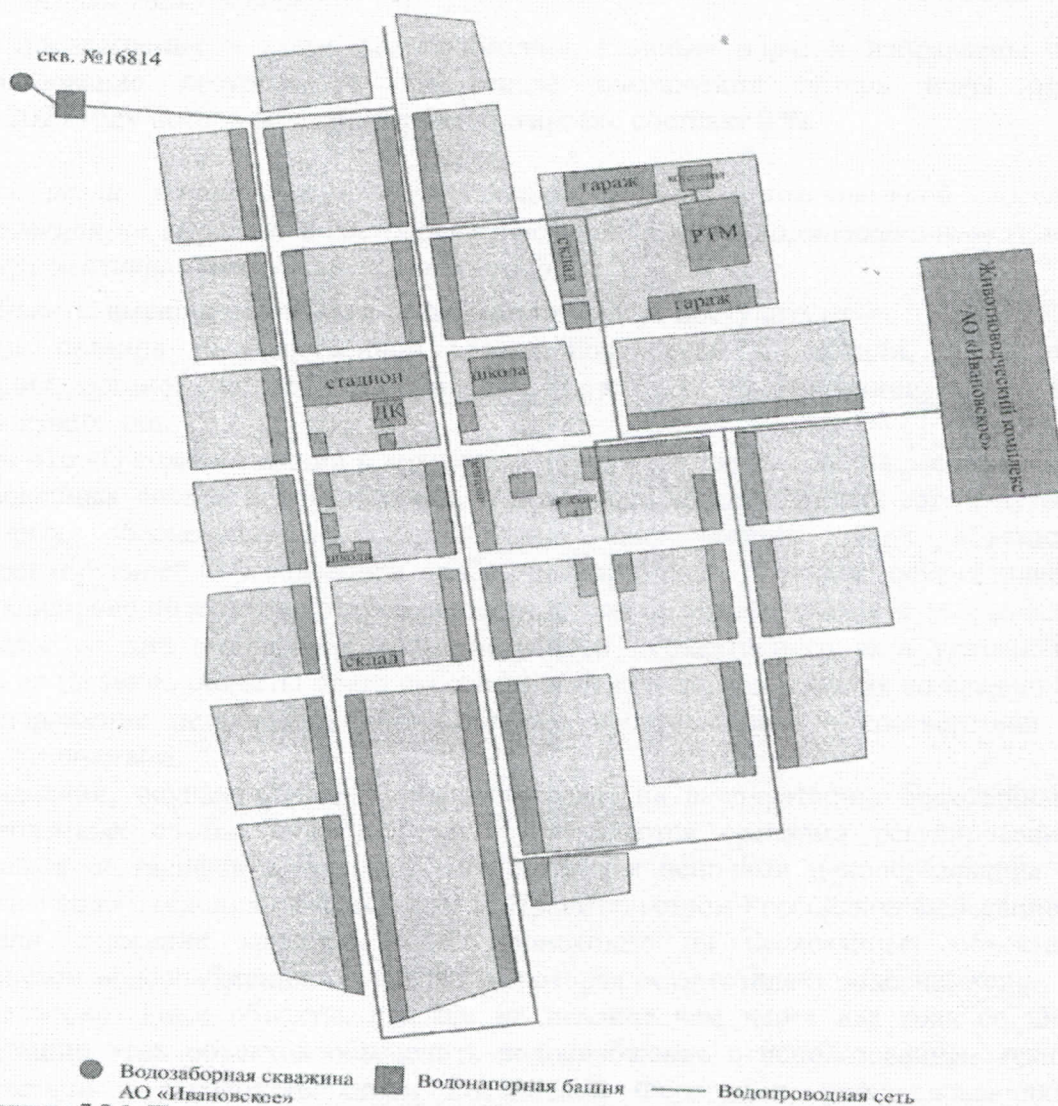
Рисунок 7.2.1. План территории АО «Ивановское» с наложением сетей водоснабжения и водоотведения (с. Ивановка)
