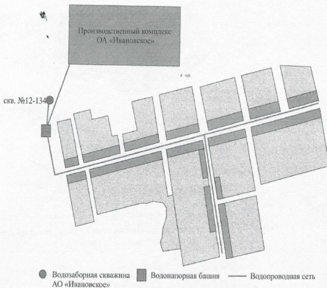
Рисунок 7.2.3. План территории АО «Ивановское» с наложением сетей водоснабжения и водоотведения (с. Грушевка)
